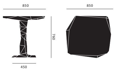
1 leg table
